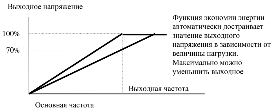
Выходная характеристика для режима экономии энергии.
